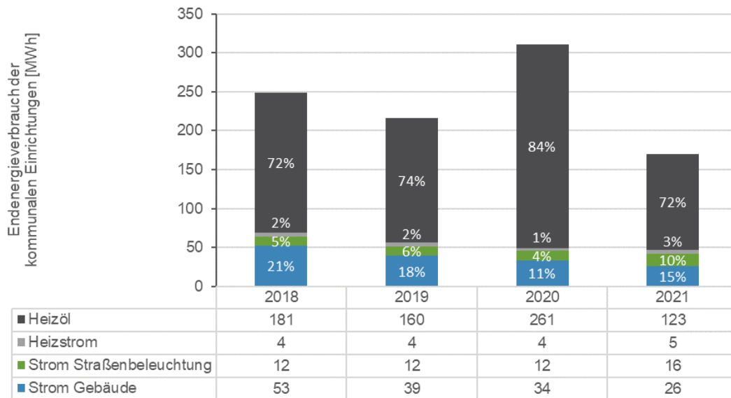
Abbildung 47 Verlauf des kommunalen Endenergieverbrauchs, 2018 – 2021
