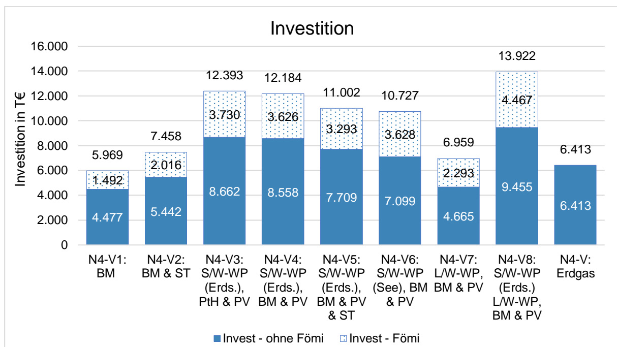
Abbildung 79 Investitionskosten WN 4 Variante 1-9
