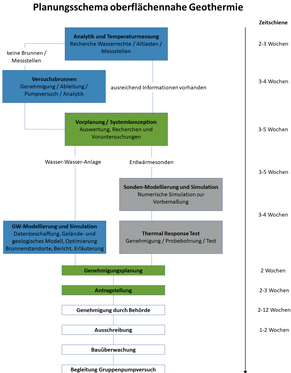
Abbildung 105 Planungsschema für oberflächennahe Geothermie 60
