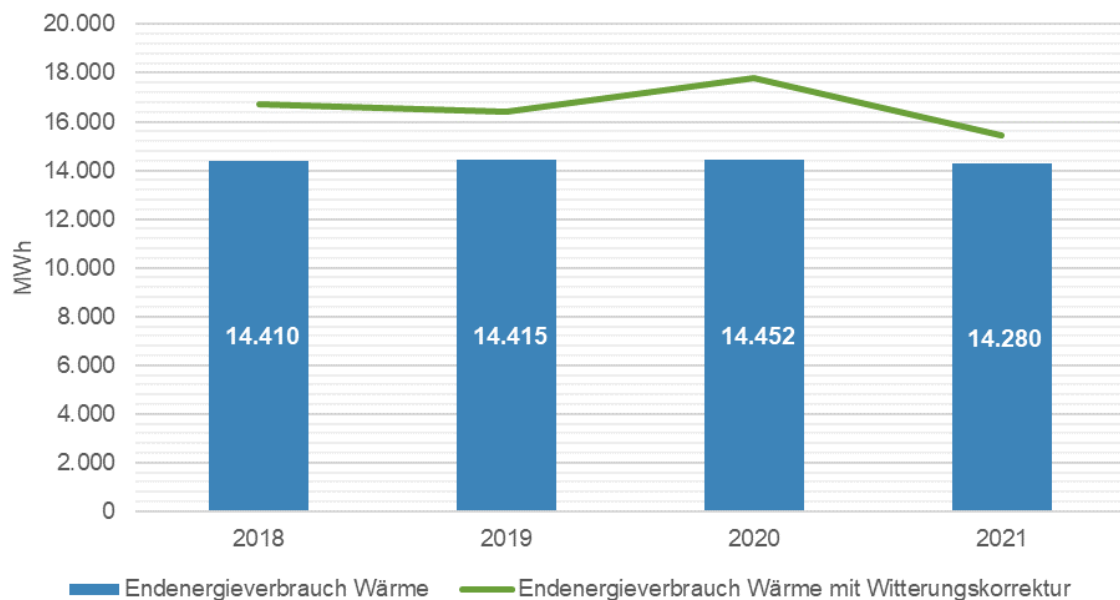
Abbildung 43 Tatsächlicher und witterungsbereinigter Endenergieverbrauch der Wärmeversorgung (mit Heizstrom), 2018 – 2021
