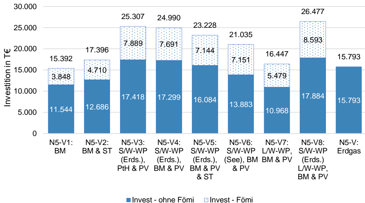
Abbildung 84 Investitionskosten WN 5 Variante 1-9
