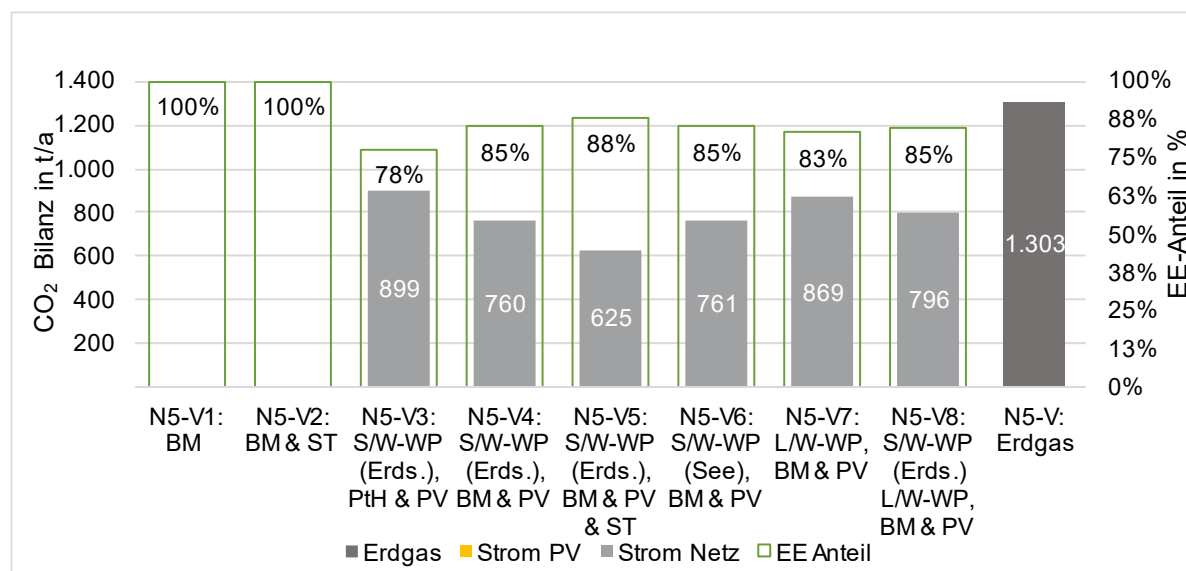
Abbildung 74 CO 2 -Bilanz WN 5, Variante 1-9 & EE-Anteil
