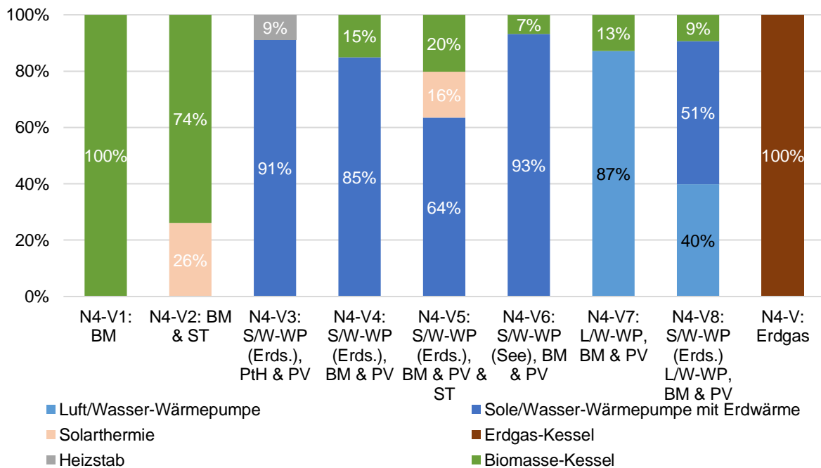
Abbildung 78 Verteilung Wärmeerzeuger WN 4 Variante 1-9
