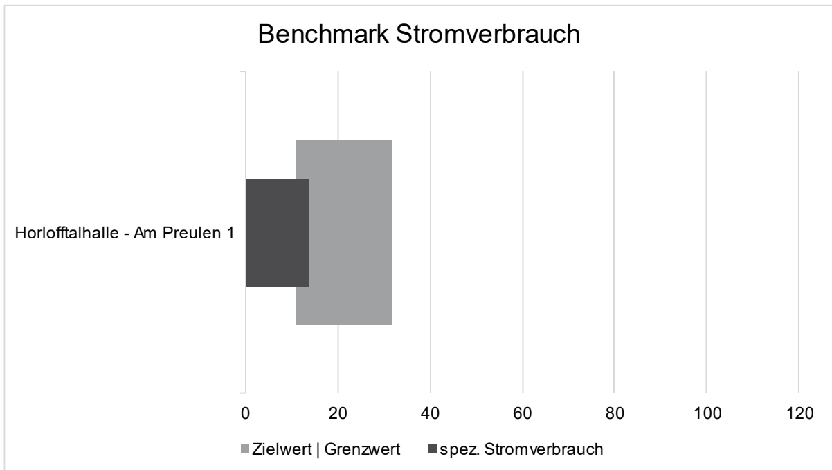
Abbildung 21 Strombenchmark in [kWh/m²] der kommunalen Gebäude 2019-2022
