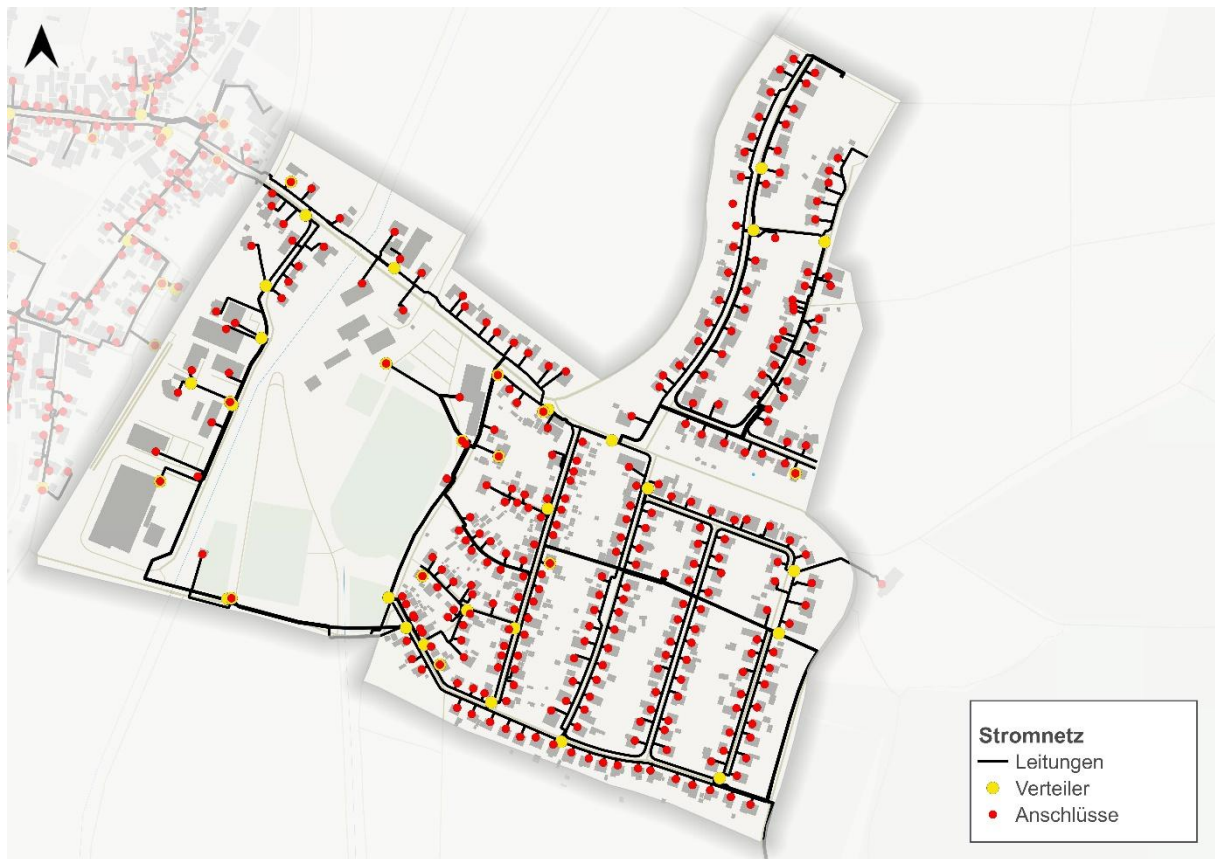
Abbildung 22 Stromnetz inklusive Anschlüsse und Verteiler in Echzell Wohngebiet
