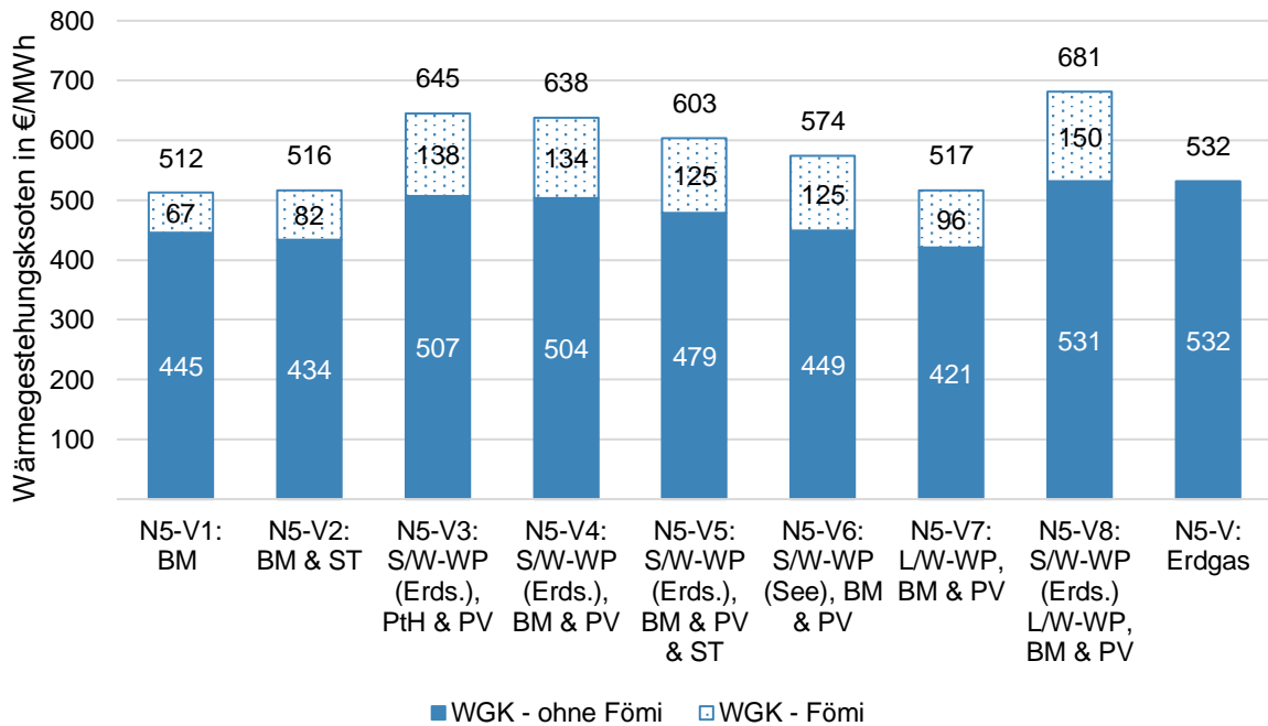
Abbildung 86 Wärmegestehungskosten für WN 5 Variante 1-9
