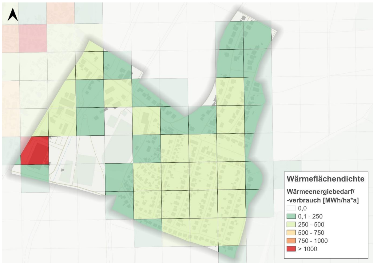
Abbildung 60 Wärmeflächendichte der georeferenzierten Gebäude einer jeden Rasterzelle in Echzell Wohngebiet
