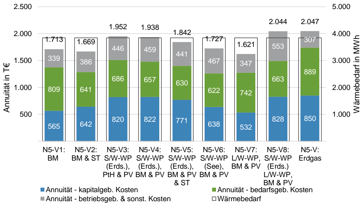
Abbildung 85 Annuität nach Förderung für WN 5 Variante 1-9 & Wärmeerzeugung p.a. in MWh
