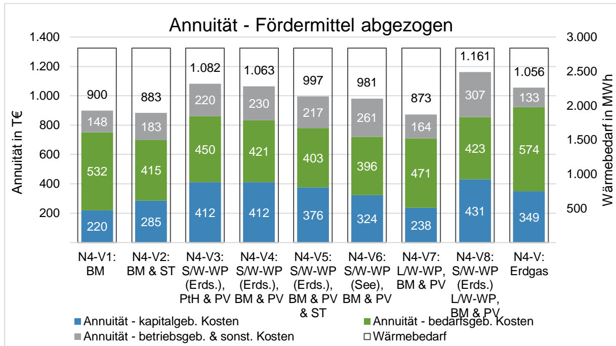
Abbildung 80 Annuität nach Förderung für WN 4 Variante 1-9 & Wärmeerzeugung p.a. in MWh
