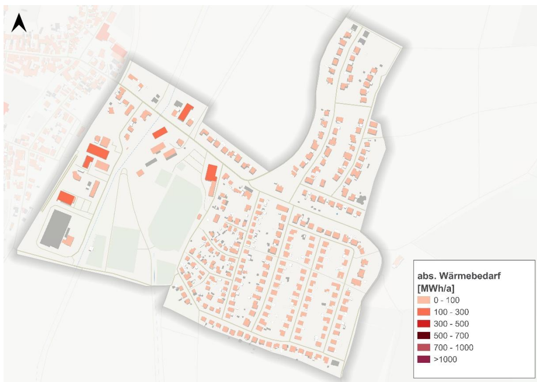
Abbildung 16 Absoluter Wärmebedarf in Echzell Wohngebiet
