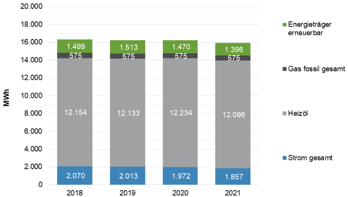
Abbildung 108 Endenergieverbrauch nach Energieträgern 2018 – 2021
