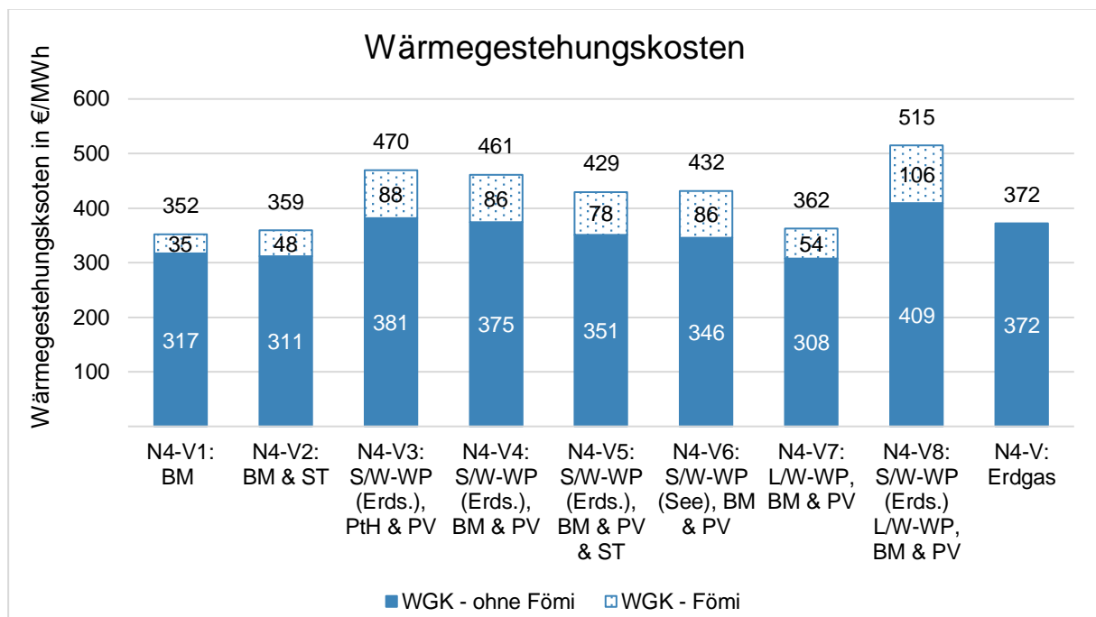
Abbildung 81 Wärmegestehungskosten für WN 4 Variante 1-9
