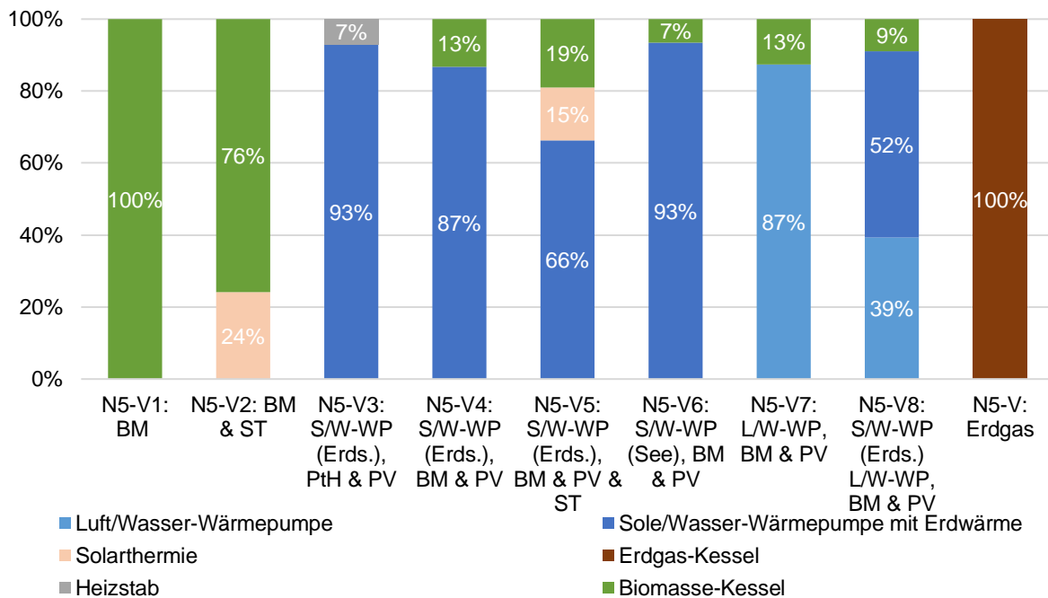
Abbildung 83 Verteilung Wärmeerzeuger WN 5 Variante 1-9
