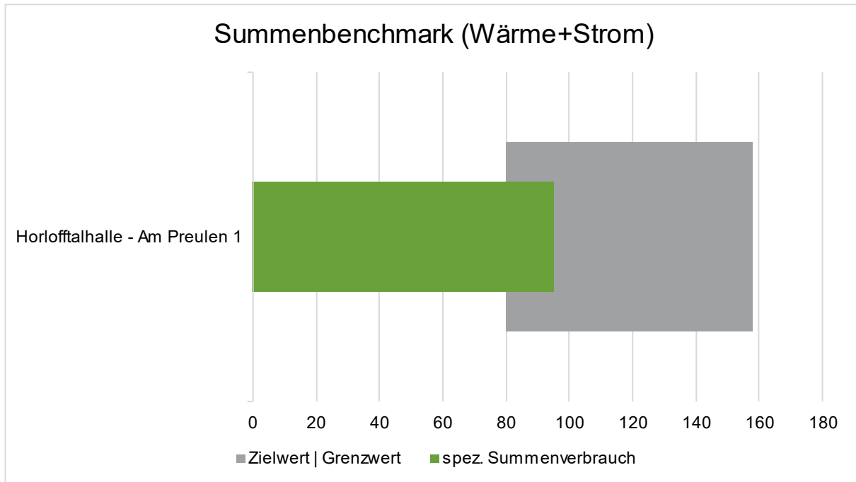
Abbildung 19 Summenbenchmark in [kWh/m²] der kommunalen Gebäude 2019-2022
