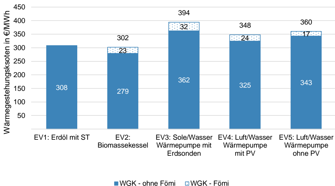
Abbildung 76 Wärmegestehungskosten Einzelversorgung
