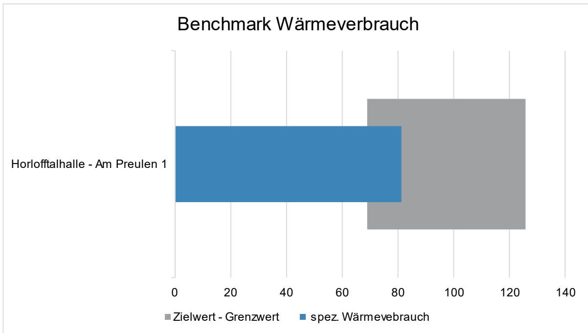
Abbildung 20 Wärmebenchmark in [kWh/m²] der kommunalen Gebäude 2019-2022
